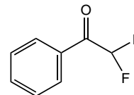
\alpha,\alpha -Difluoroacetophenone
